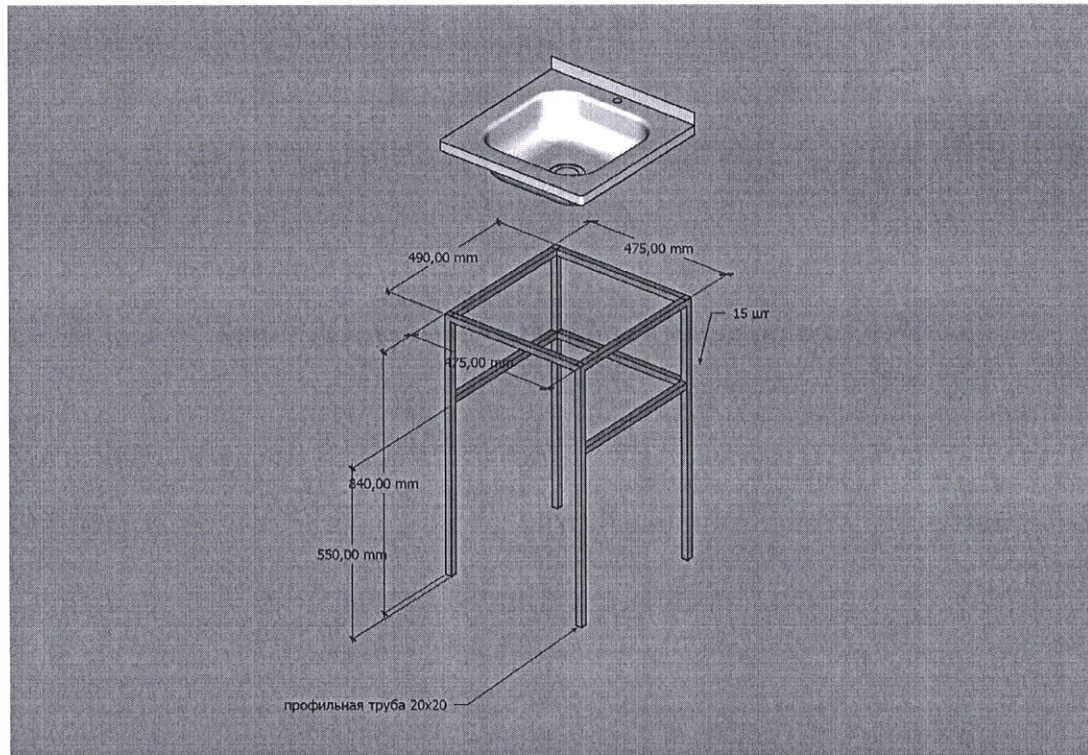
Рис. 1 Каркас-подставка для умывальника
