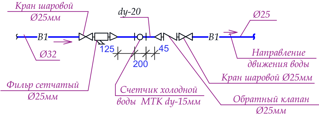
Водомерный узел ВУ-1
