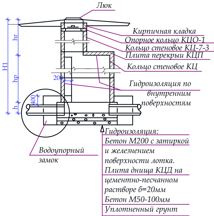
Колодец канализационный
