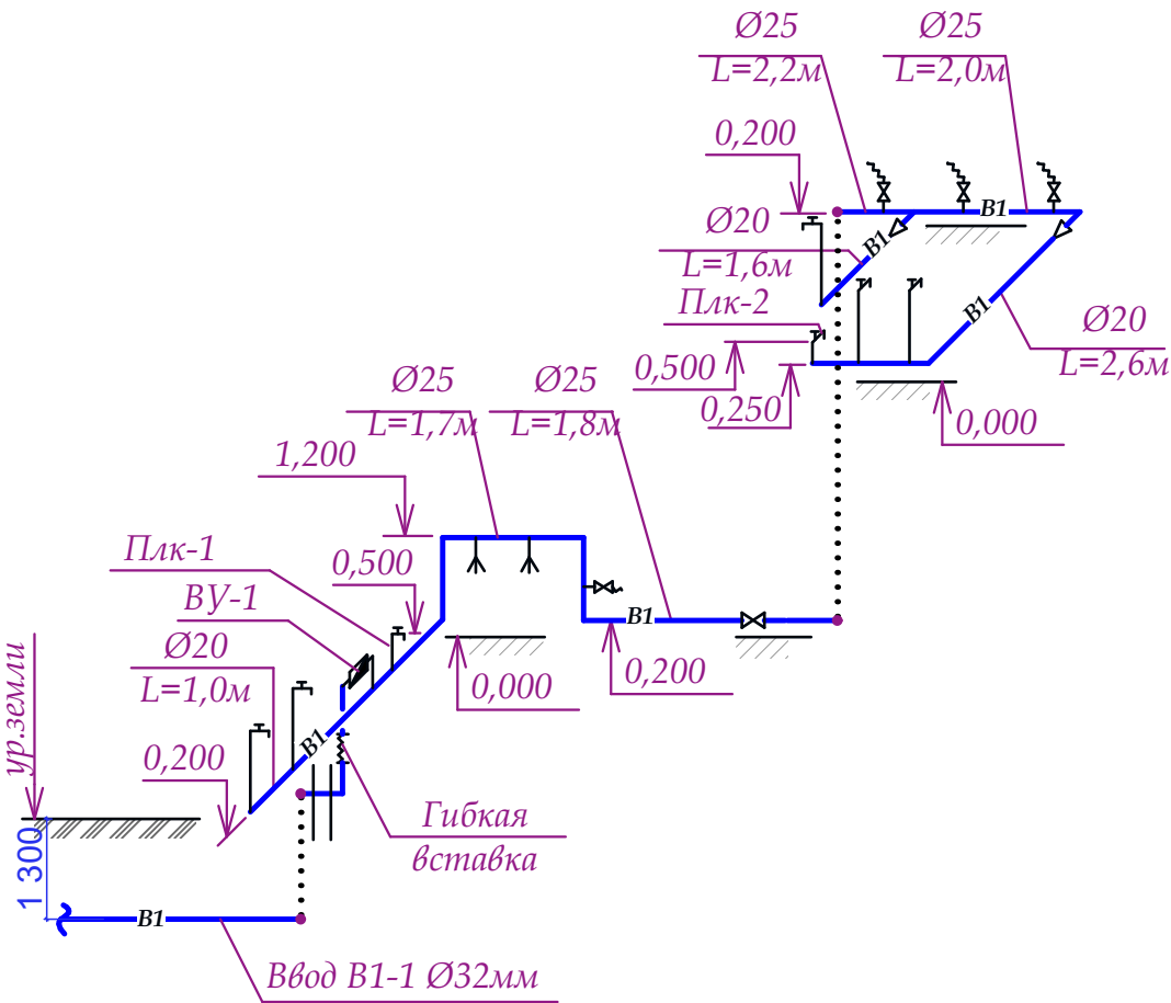
Схема сети В1.
