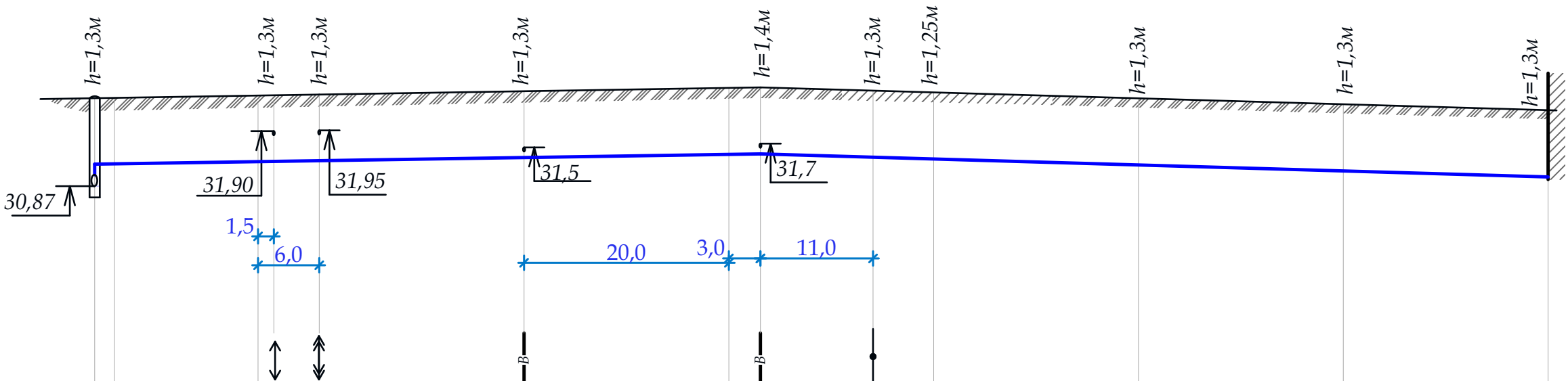
Продольный профиль В1.
