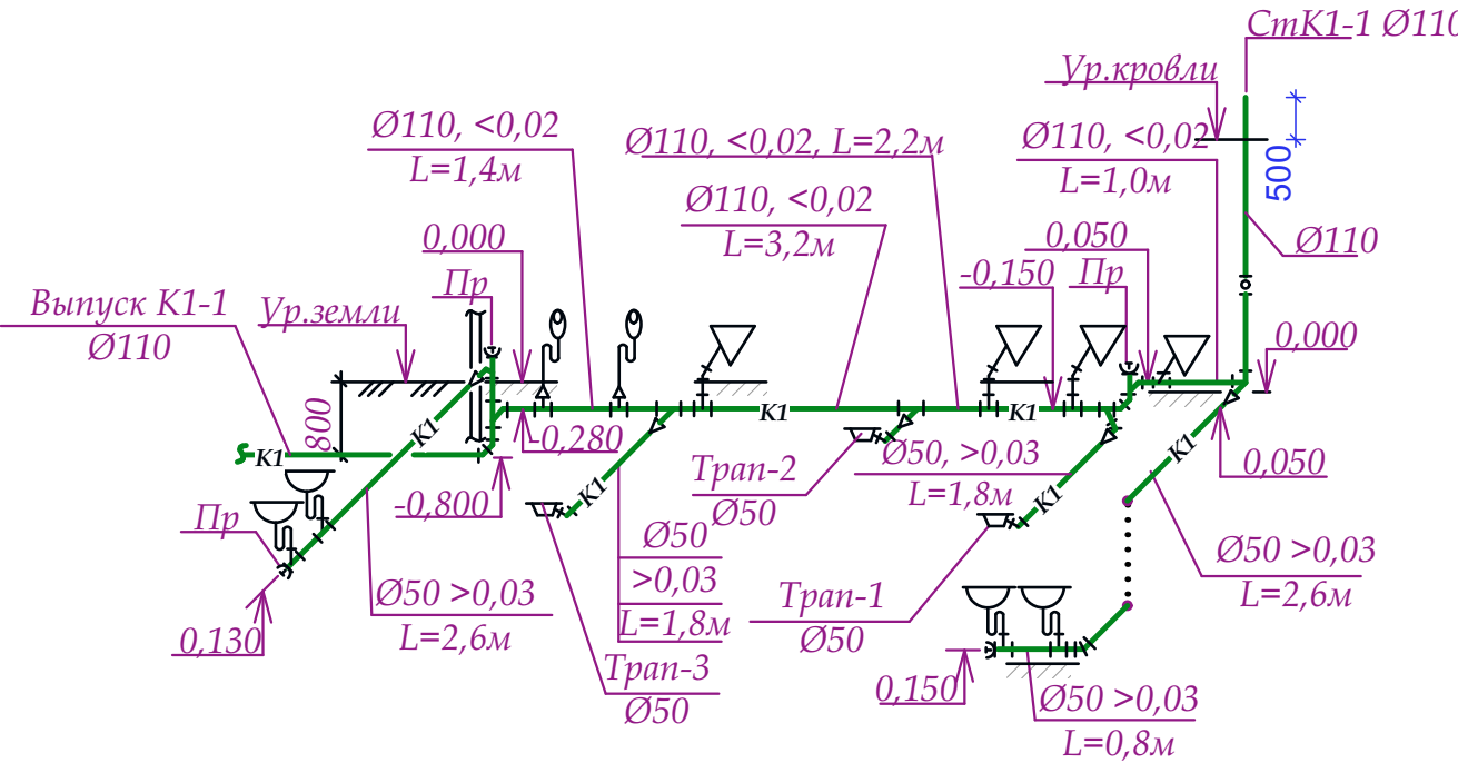
Схема сети К1.
