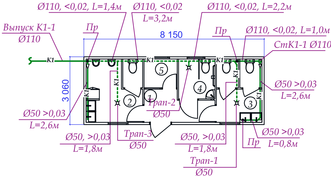
Схема сети К1.
