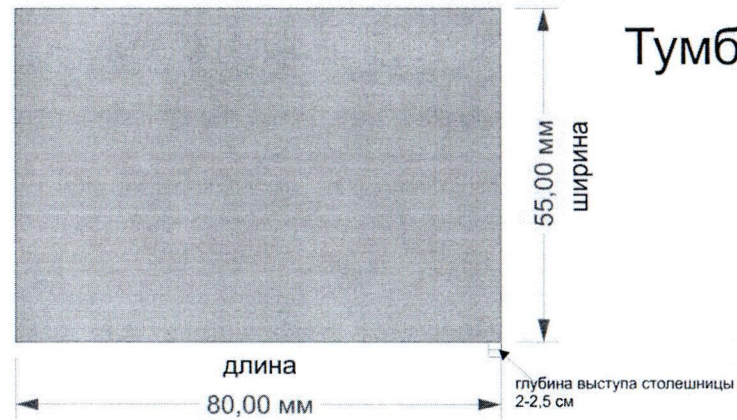
ВИД СВЕРХУ
