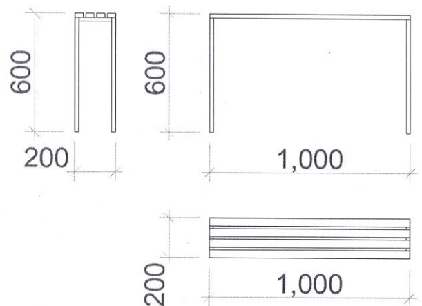
Рис. 2 Каркас-подставка для сумок
