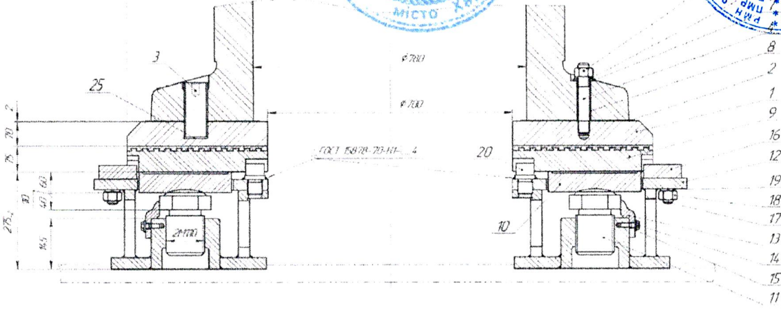
Вид на опорные болты сегменты и тарелки сняты
