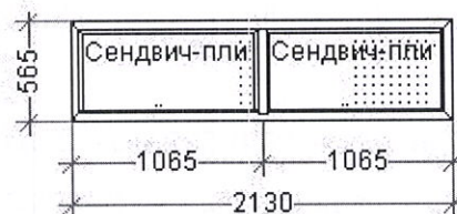
Конструкция 22 – 2130*565 мм – 1 шт.
