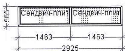
Конструкция 25 – 2925*565 мм – 1 шт.
