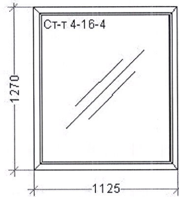
Конструкция 30 – 1125*1270 мм – 2 шт.
