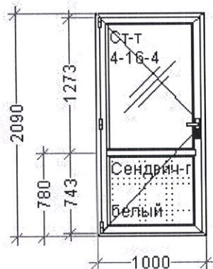
Конструкция 15 – 1000*2090 мм – 1 шт.
