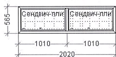
Конструкция 36 – 2020*565 мм – 1 шт.
