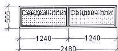
Конструкция 26 – 2480*565 мм – 1 шт.
