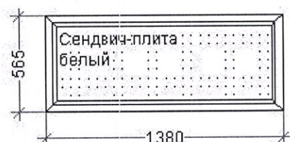
Конструкция 6 – 1380*565 мм – 1 шт.
