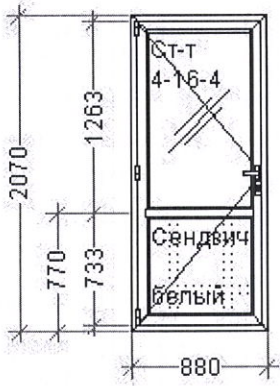
Конструкция 27 – 880*2070 мм – 1 шт.
