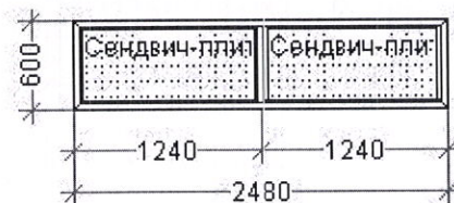
Конструкция 4 – 2480*600 мм – 1 шт.
