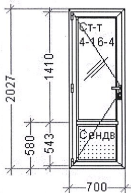
Конструкция 37 – 700*2027 мм – 1 шт.
