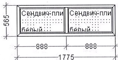
Конструкция 17- 1775*565 мм – 1 шт.
