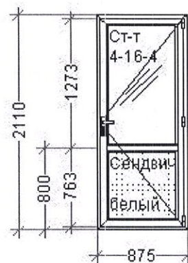
Конструкция 40 – 875*2110 мм – 1 шт.
