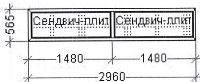
Конструкция 3 – 2960*565 мм – 1 шт.
