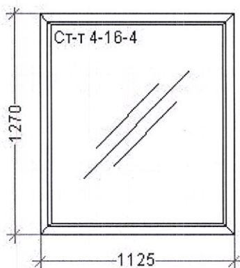
Конструкция 41 – 1125*1270 мм – 1 шт.
