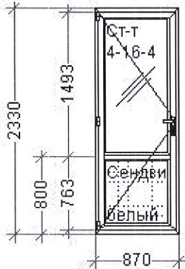
Конструкция 49 – 870*2330 мм – 1 шт.
