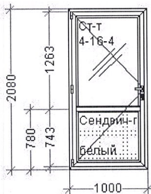
Конструкция 1 – 1000*2080 мм – 1 шт.
