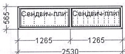
Конструкция 5 – 2530*565 мм – 1 шт.
