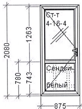
Конструкция 19- 875*2080 мм – 1 шт.
