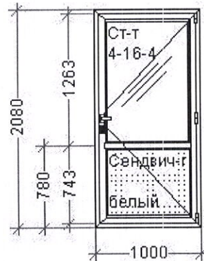
Конструкция 2 – 1000*2080 мм – 1 шт.
