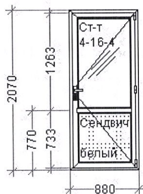
Конструкция 23-880*2070 мм – 1 шт.
