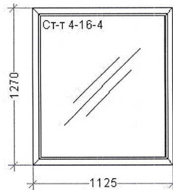
Конструкция 34 – 1125*1270 мм 1 шт.
