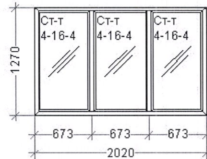
Конструкция 48 – 2020*1270 мм – 1 шт.
