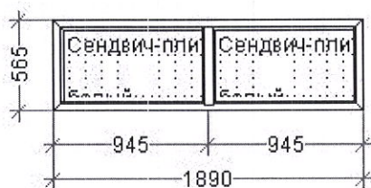
Конструкция 35 – 1890*565 мм – 1 шт.
