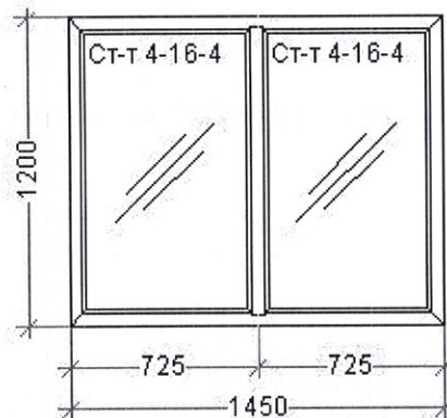
Конструкция 24 – 1450*1200 мм – 1 шт.
