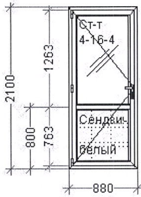
Конструкция 45 – 880*2100 мм – 1 шт.
