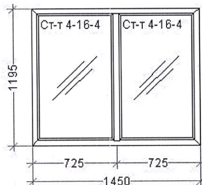
Конструкция 20 – 1450*1195 мм – 1 шт.
