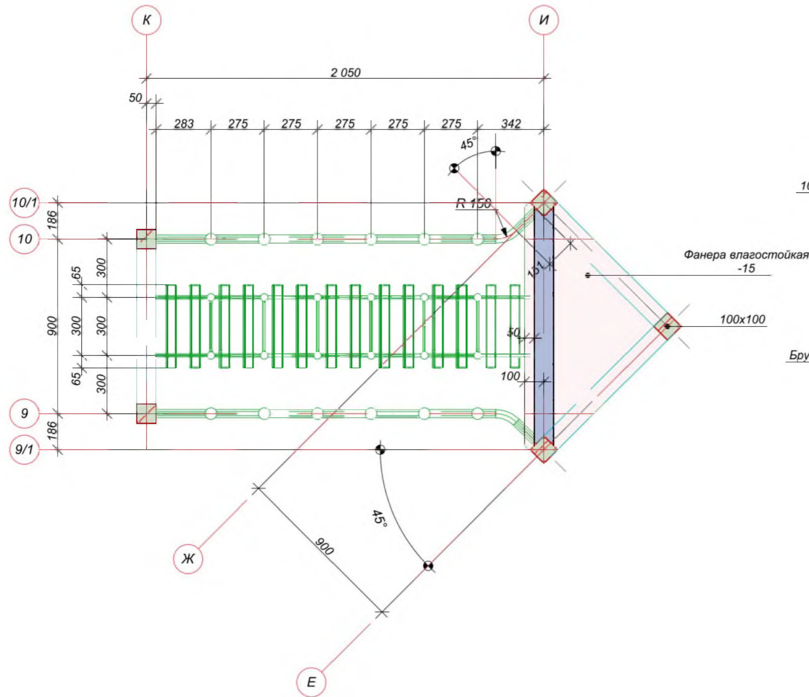
План М 1:50
