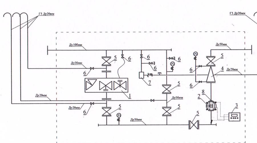
Функциональная схема ШГРП
