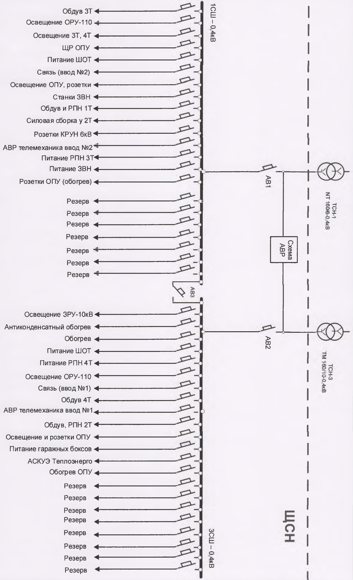
СХЕМА собственных нужд ПС «Бендеры Южная – 110/35/10/6 кВ»
