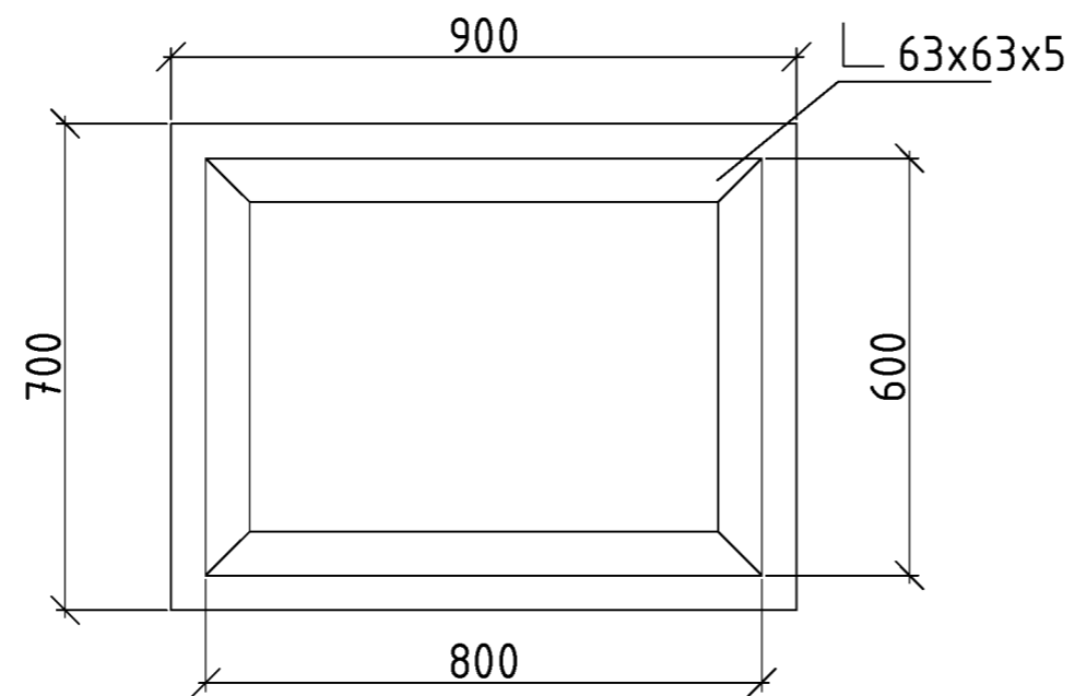
Вид сверху
